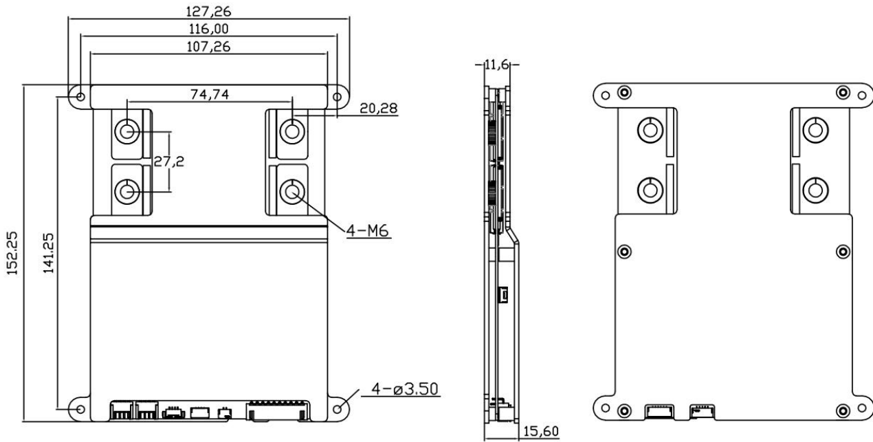
JK-BxA8S-20P 外形尺寸
