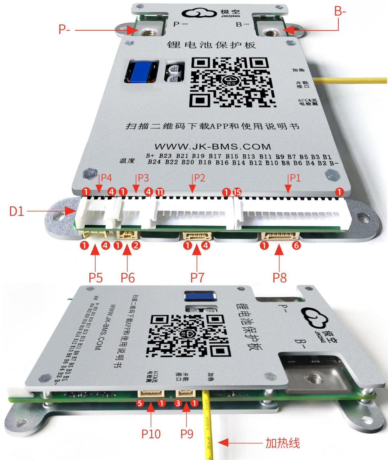
JK-BD6AxxS-6PT/8PT连接器示意图
