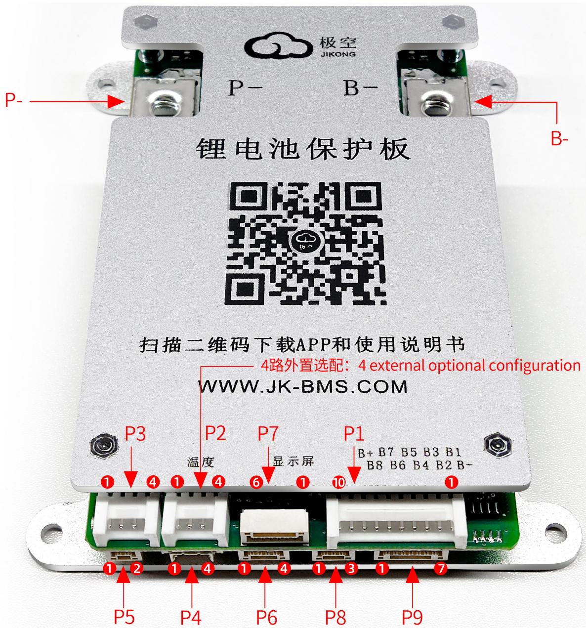
JK-BD4A8S-4P/6P 连接器示意图
