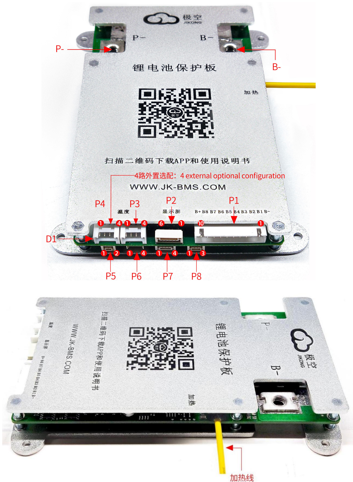
JK-B1A8S-10P 连接器示意图
