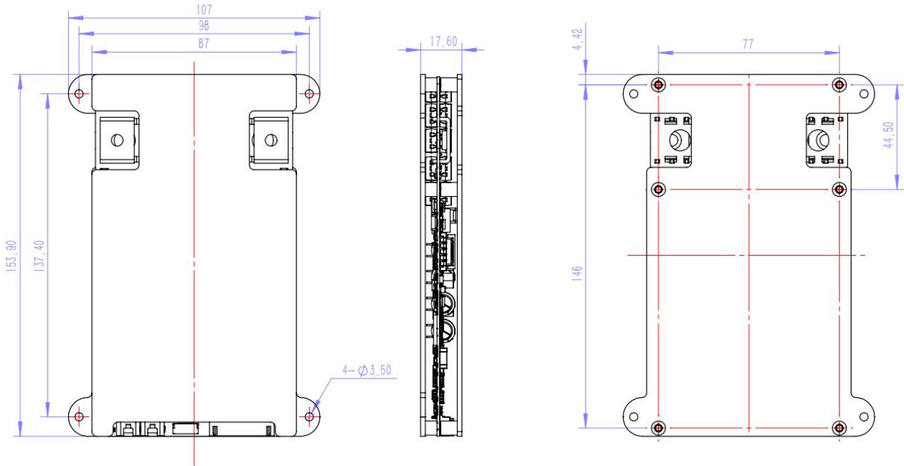
JK-B1A8S-10P 外形尺寸
