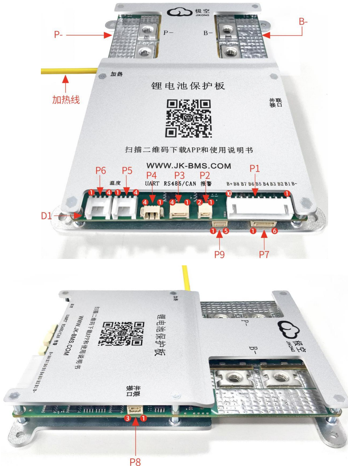
JK-BxA8S-20P 连接器示意图
