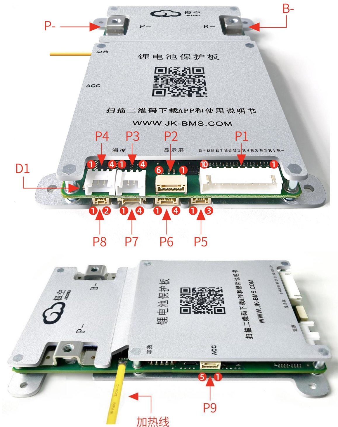
JK-B1A8S-10P 连接器示意图
