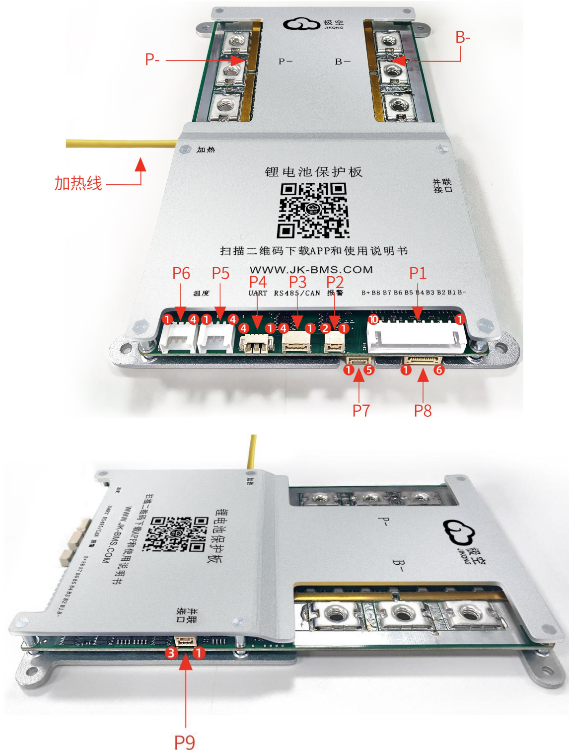
JK-B2A8S-30P 连接器示意图
