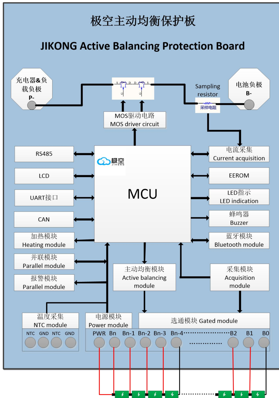
JK-BD4AxxS-6P/8P 结构框图
