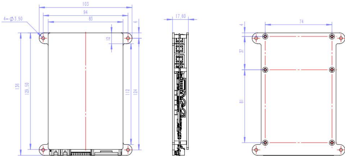
JK-BD4AxxS-6P/8P 外形尺寸
