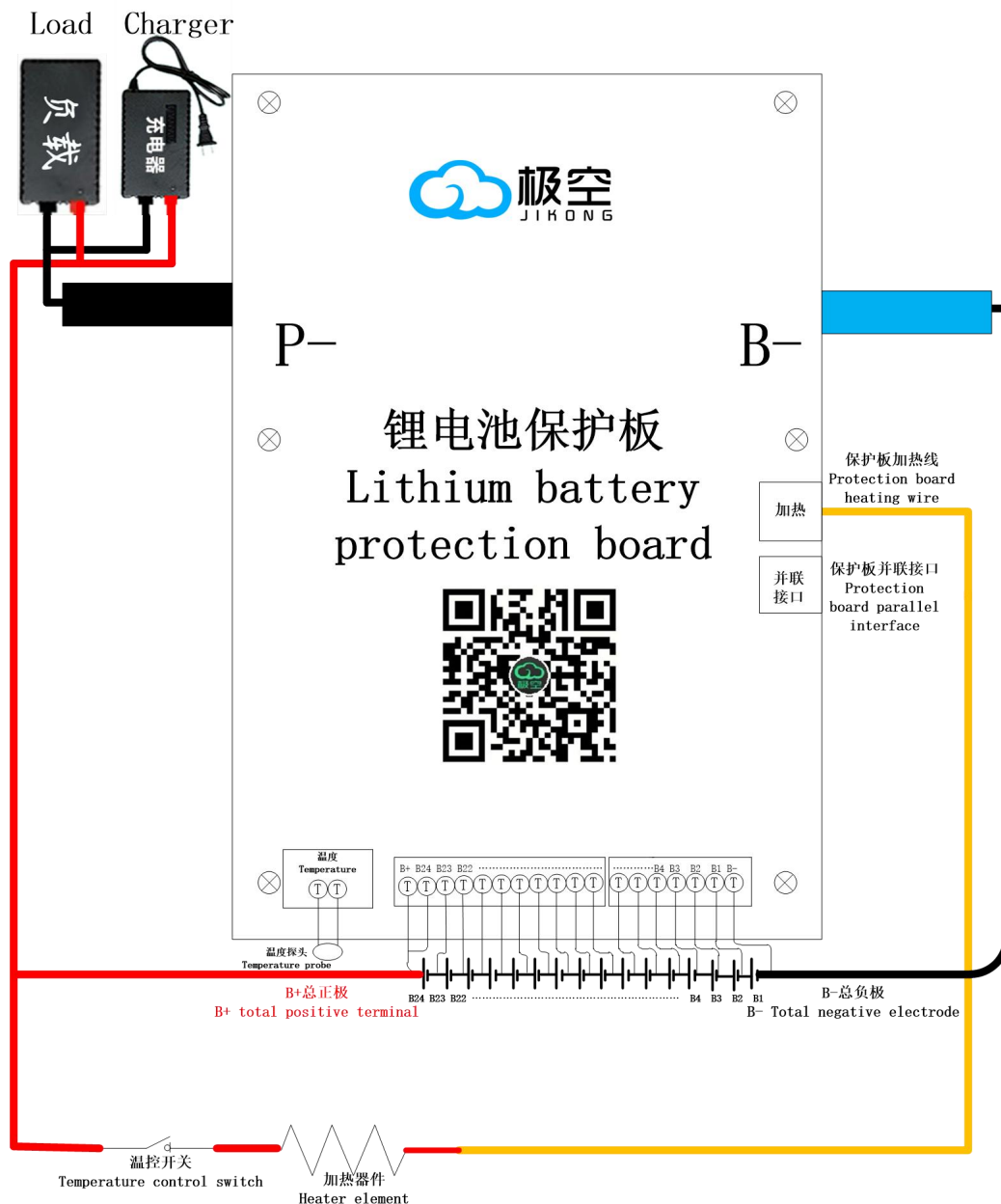
JK-BD4A24S-4P-24S接线图
