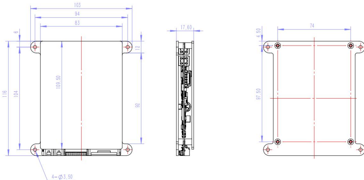
JK-BD4A24S-4P 外形尺寸
