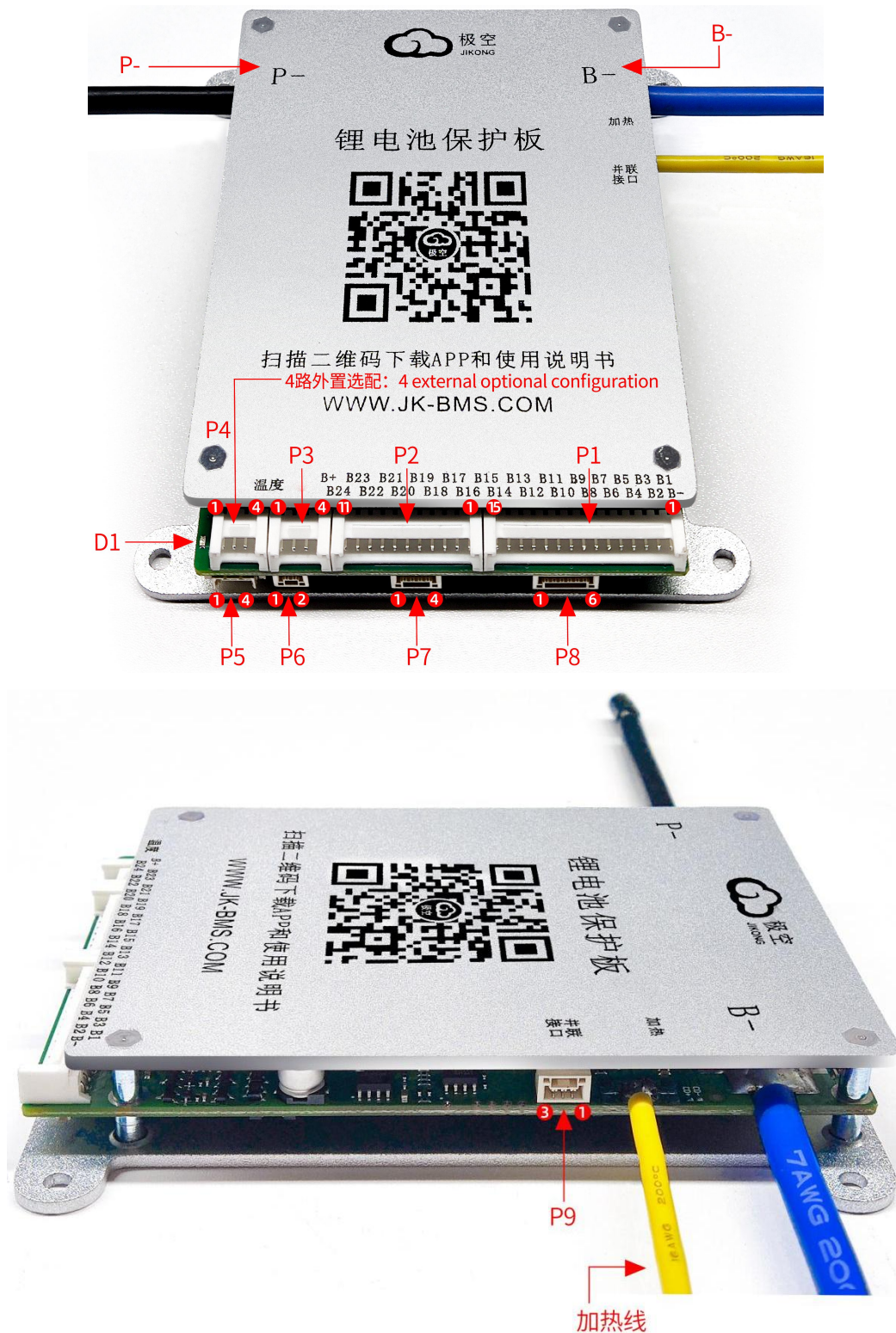
JK-BD4A24S-4P 连接器示意图
