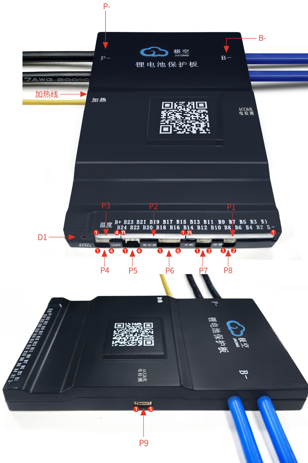
JK-BD6AXXS-10P/12P/15P/20P 连接器示意图
