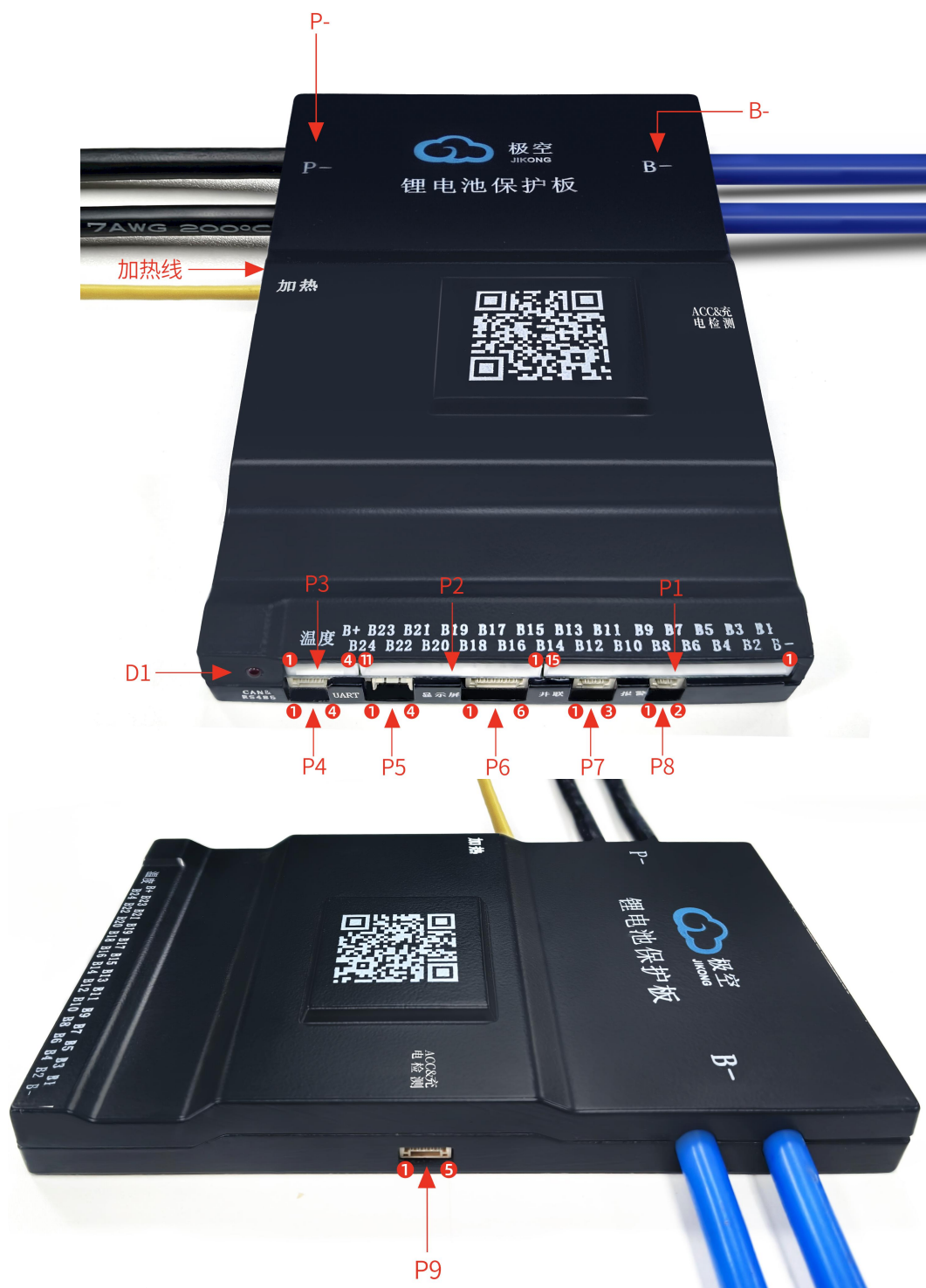
JK-BxAxxS-15P/20P 连接器示意图
