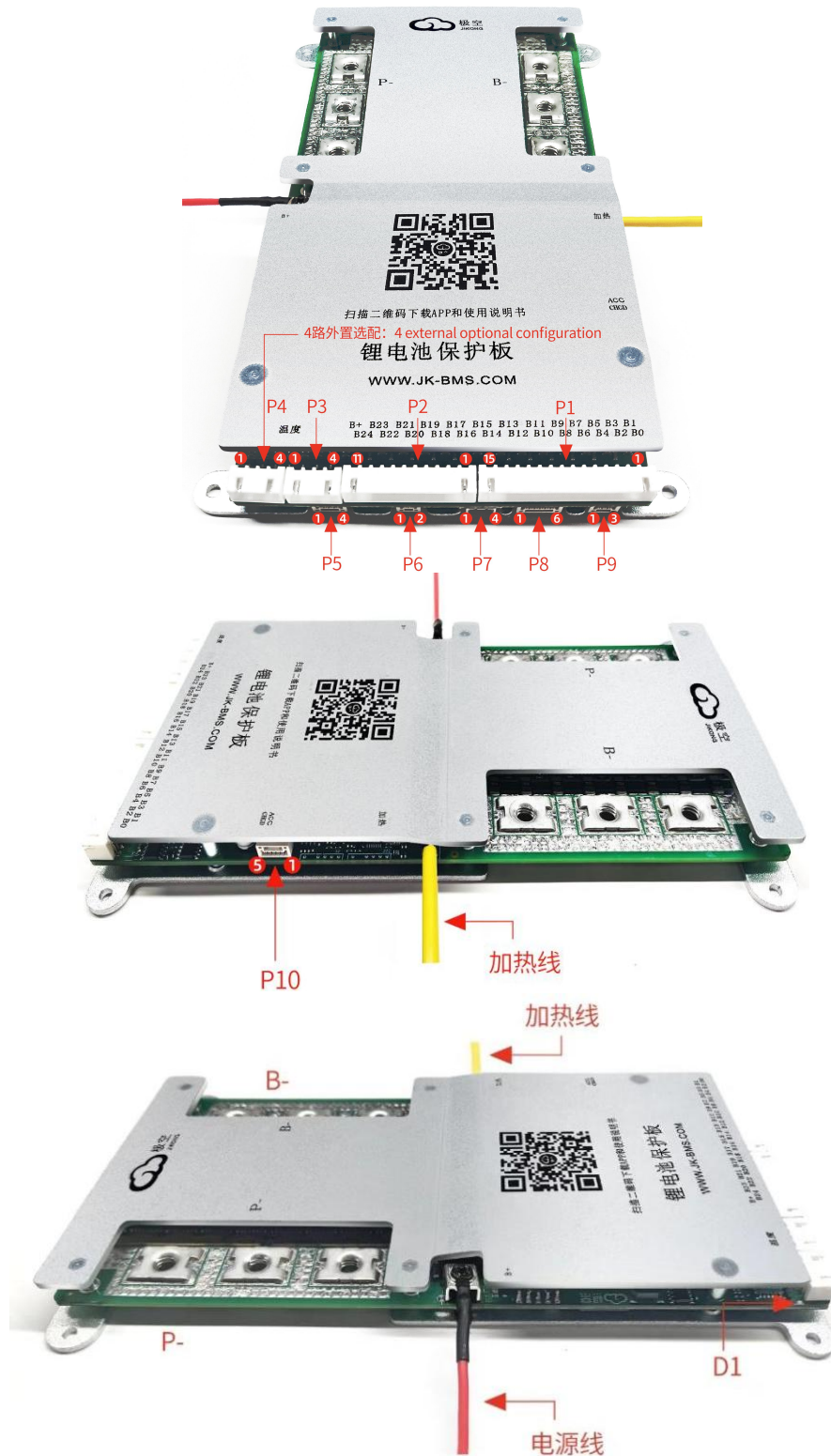
JK-B2A24S-30P 连接器示意图
