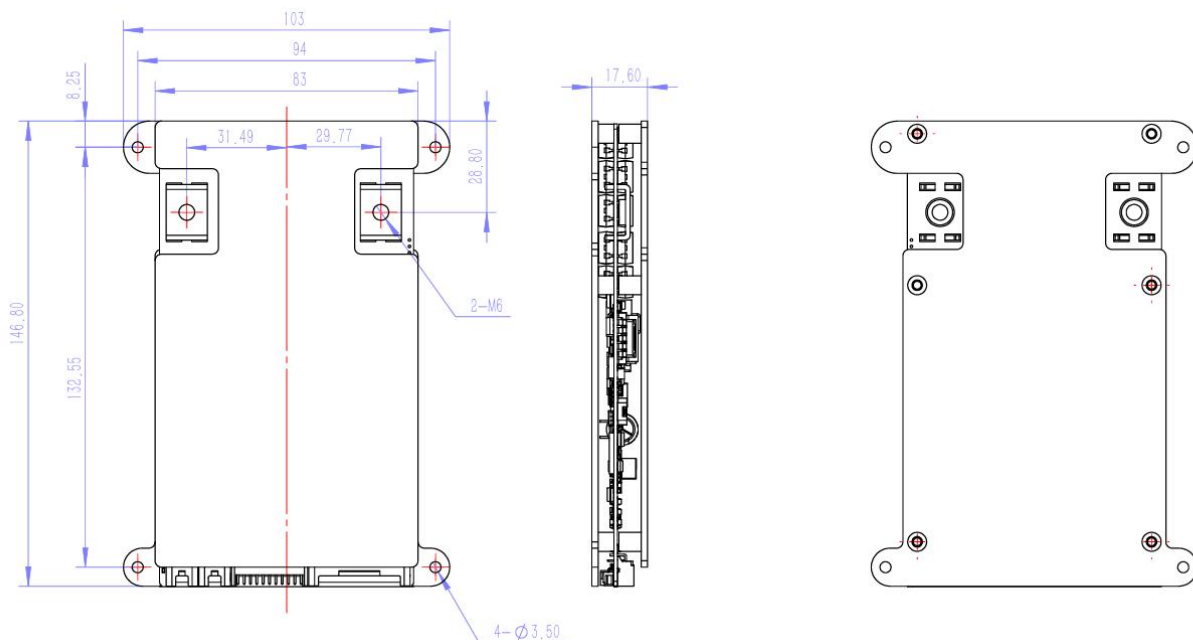
JK-BD4AxxS-10P外形尺寸
