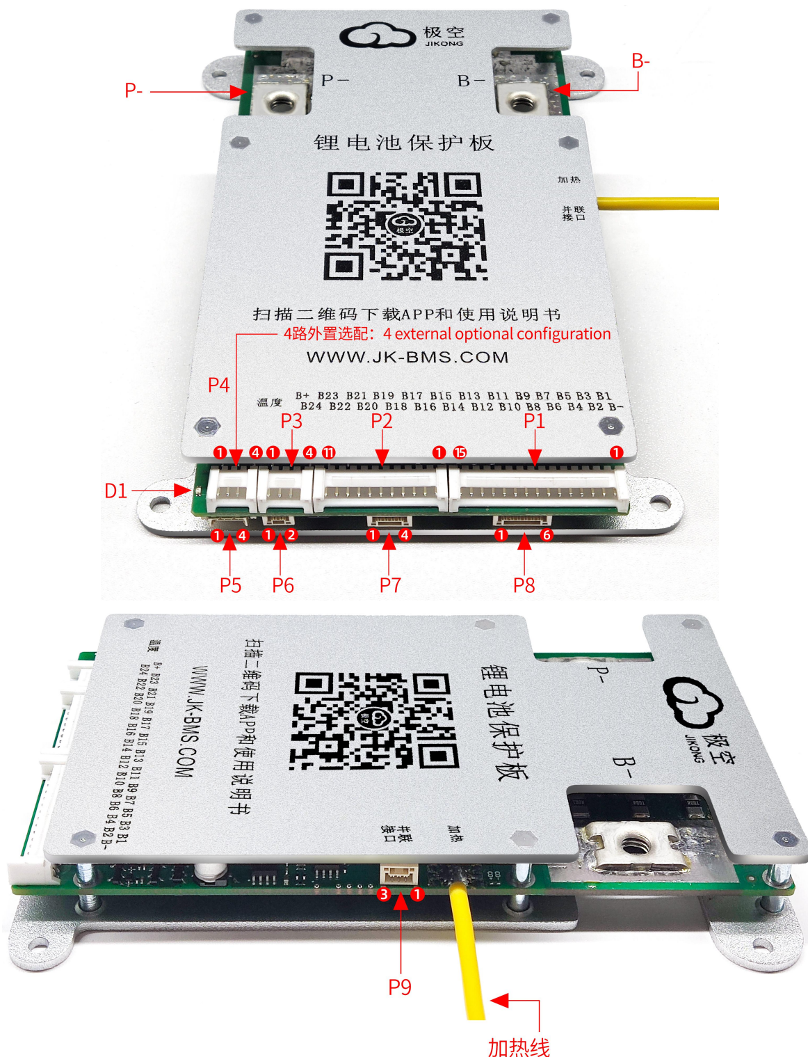
JK-BD4AxxS-10P 连接器示意图
