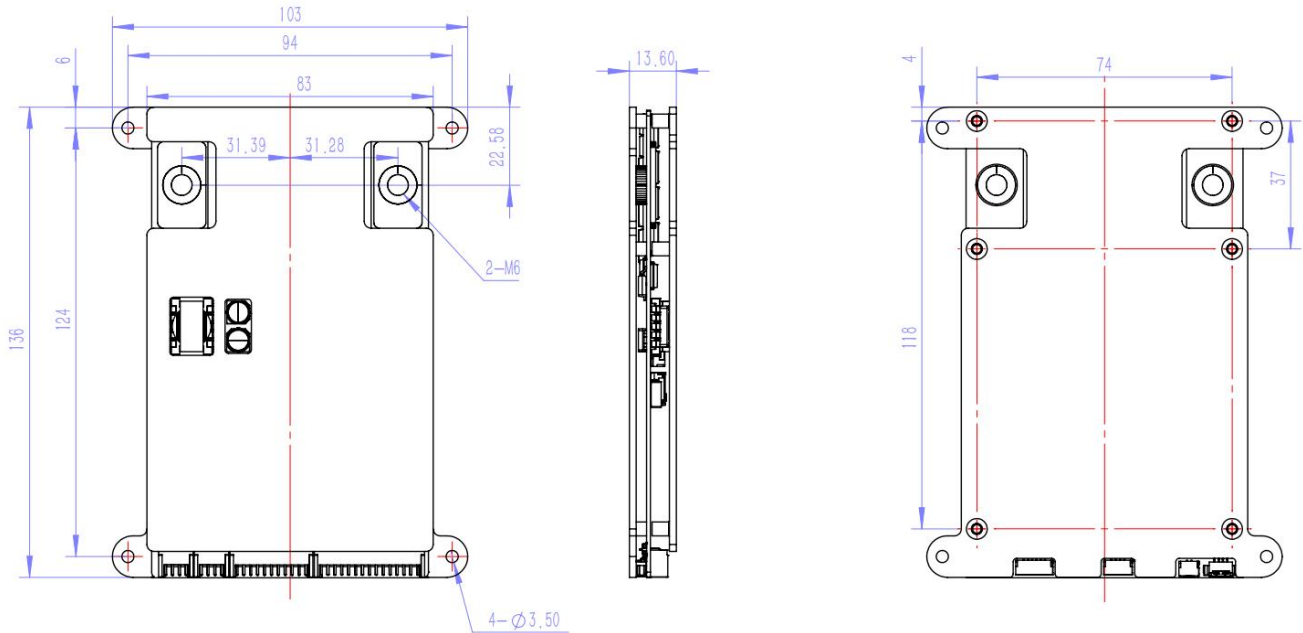
JK-BD6AxxS-8PD外形尺寸
