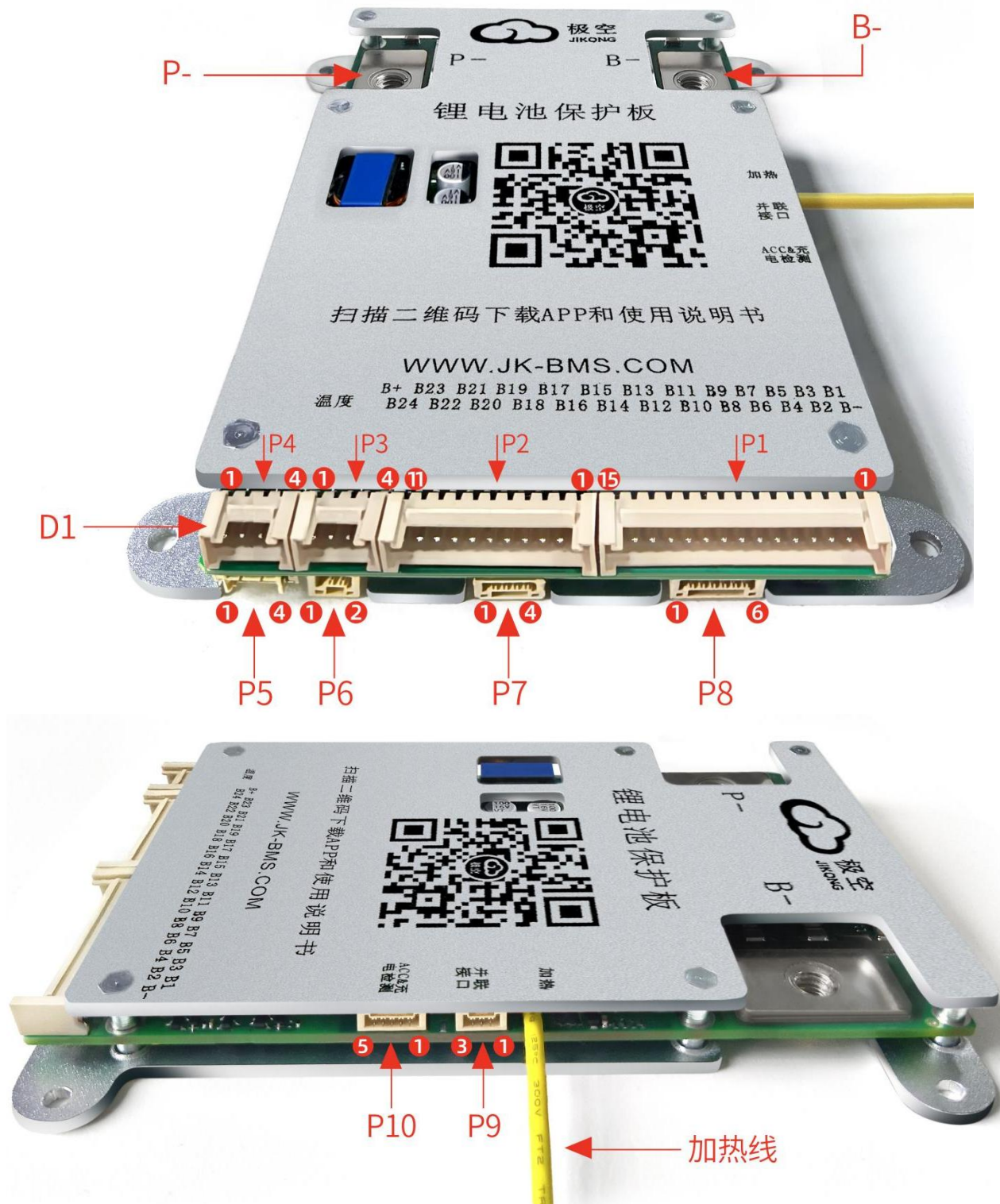
JK-BD6AxxS-8PD连接器示意图
