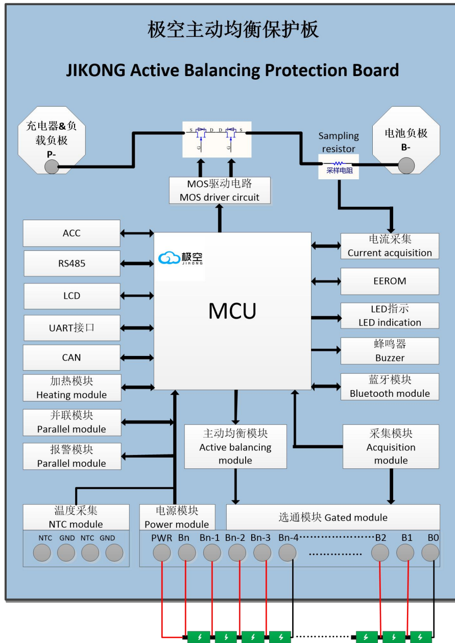
JK-BD6AxxS-8PD结构框图
