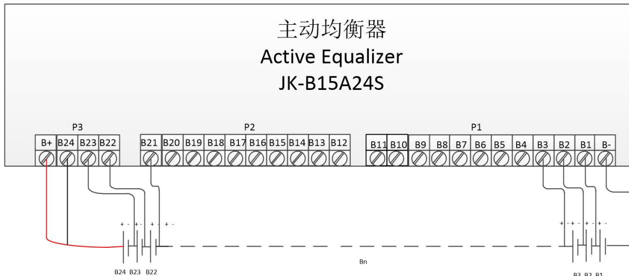
JK-B15A24S 接线图
