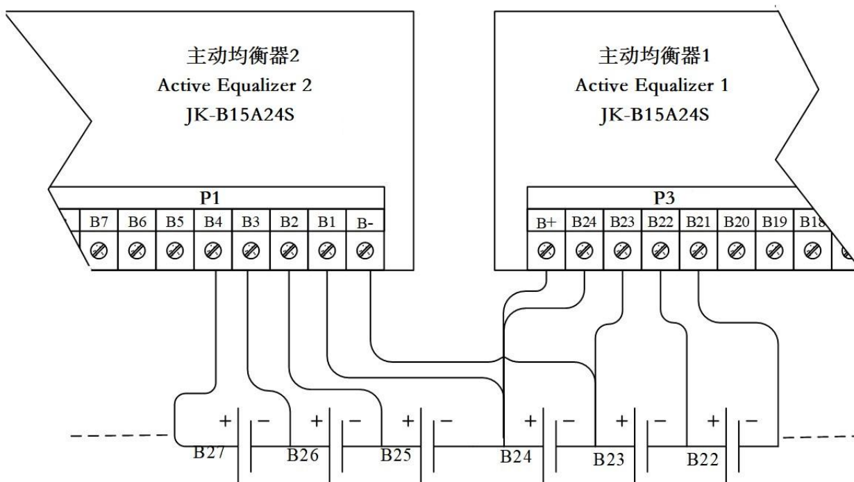
均衡器级联接线图 Equalizer Cascade Wiring Diagram
