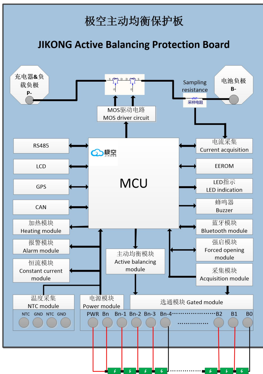
JK-QB2A8S-20P 结构框图
