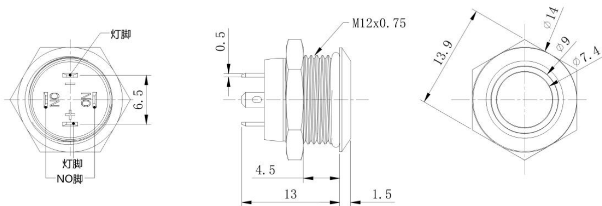
激活开关尺寸
