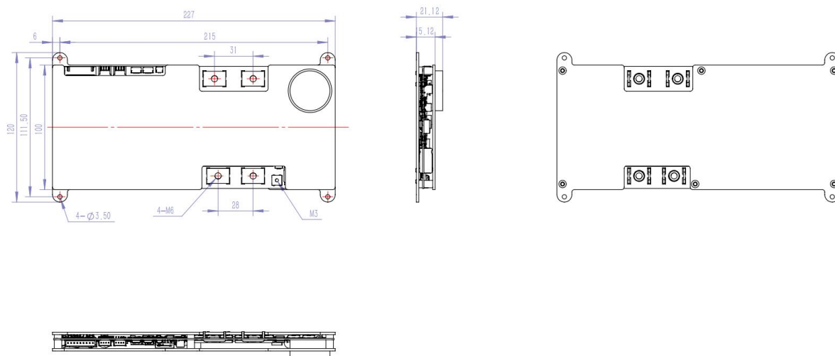
JK-QB2A8S-20P 外形尺寸
