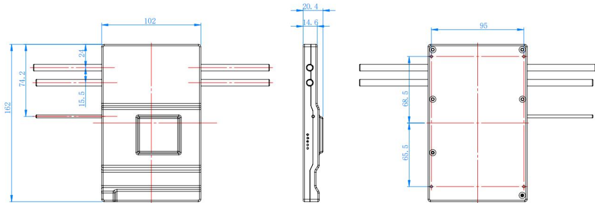
JK-BD4AxxS-10P外形尺寸
