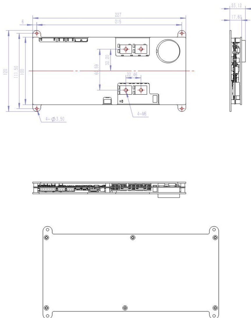
JK-QB2A8S-20P 外形尺寸
