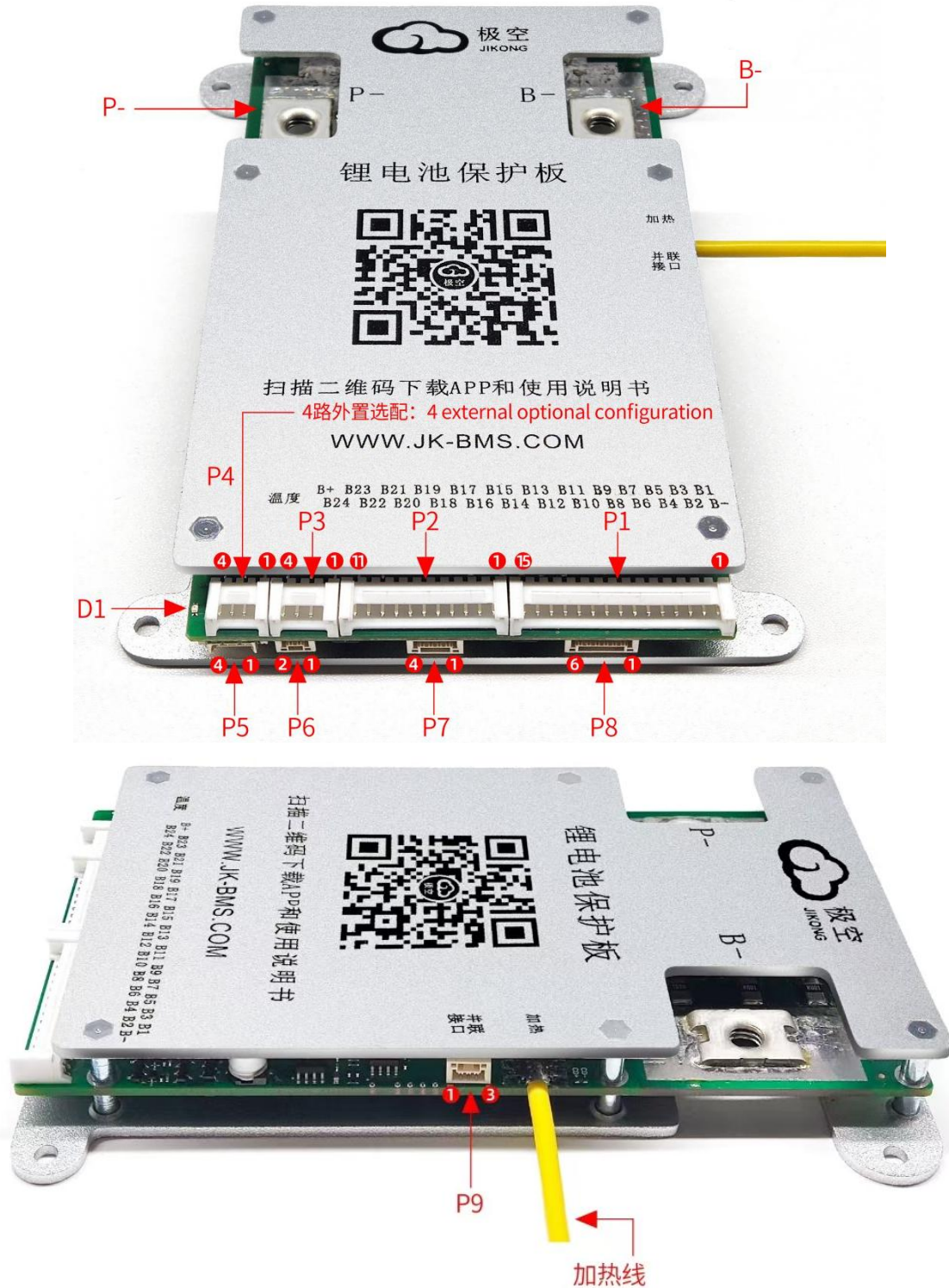
JK-BD4AxxS-10P 连接器示意图
