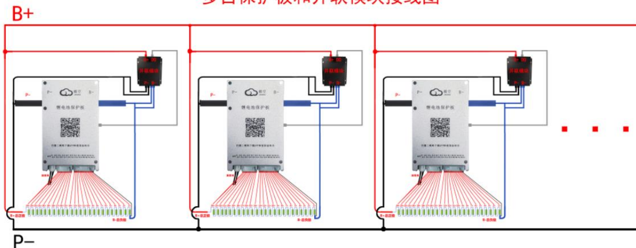
多台保护板和并联模块接线图
