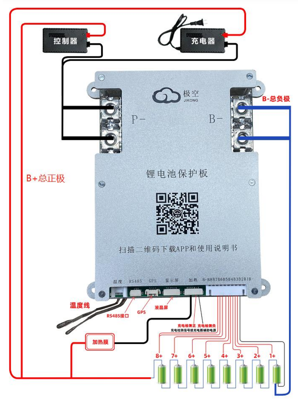
图 4 8串电池接线图示
