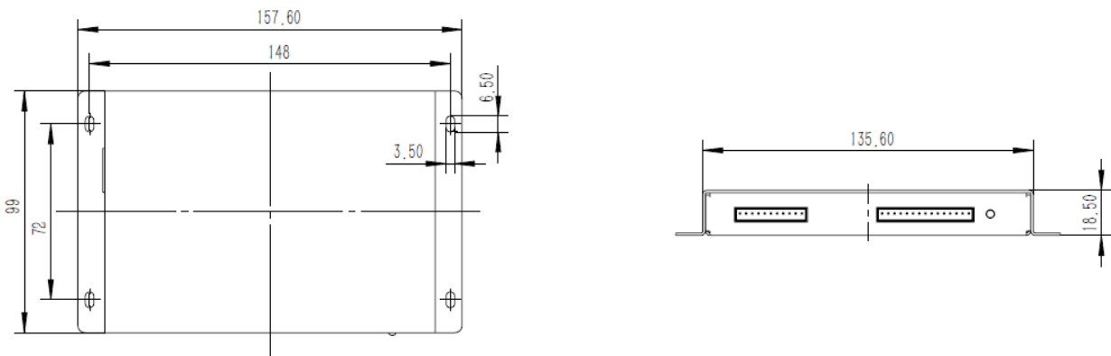
图 3 JK-B1A16STH 外形尺寸图
