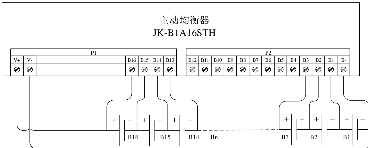
图 4 16 串电池接线图示
