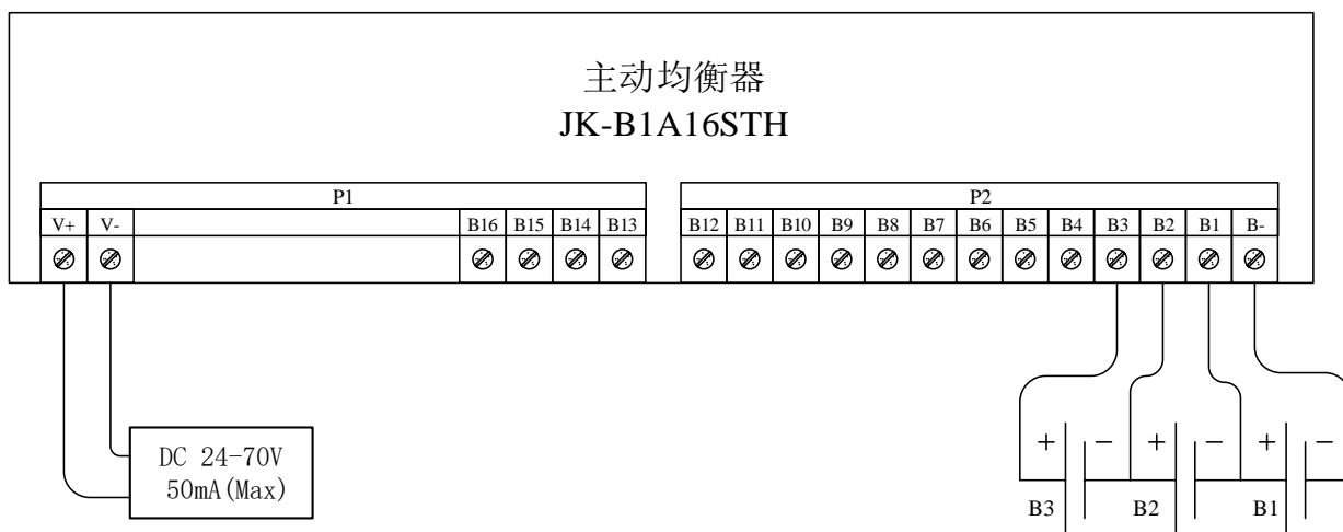
图 5 外部供电接线
