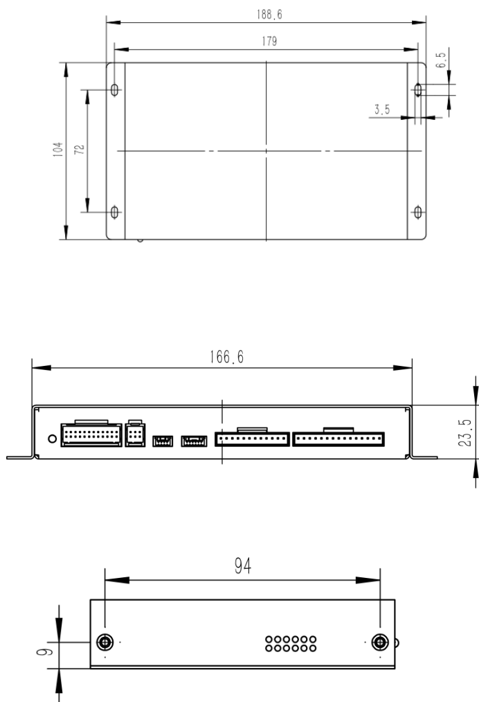
图 3 JK-B2A25S-RP 外形尺寸图
